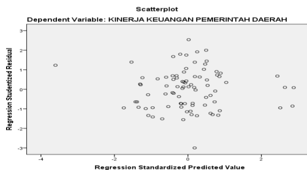
Gambar 1. Uji Heteroskedastisitas
